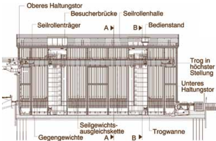
Längsschnitt
