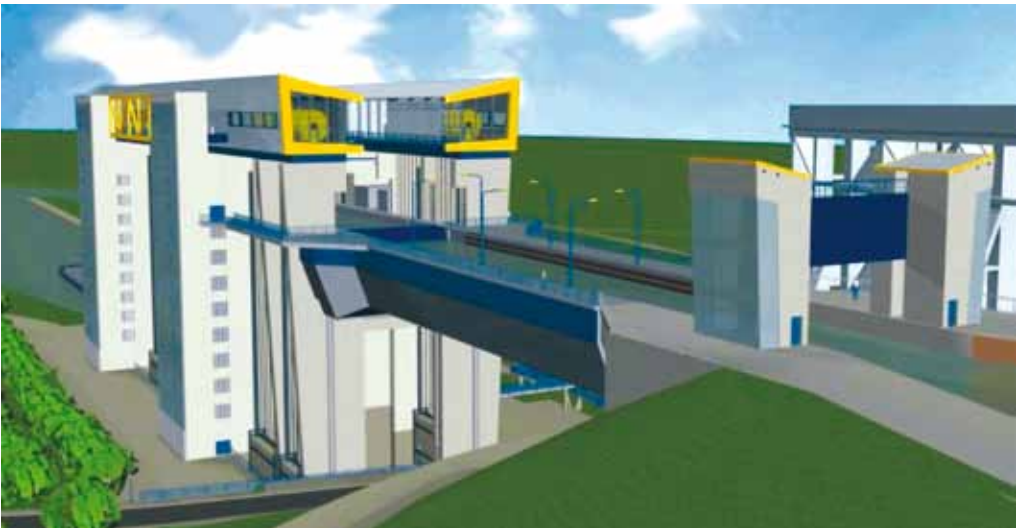
Blick von Nordwest auf das neue Schiffshebewerk und die Kanalbrücke
