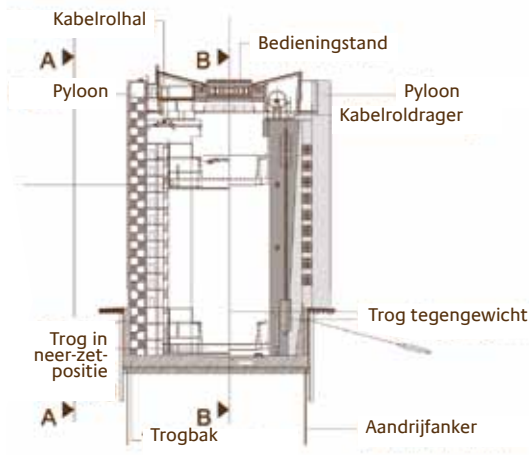
Doorsnede
